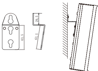
壁掛けブラケット(付属品)
