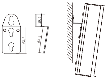
墙壁挂架 (附属品)
