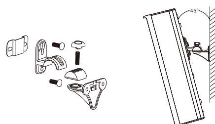
可调节角度壁挂架 (0-45° 选配)
