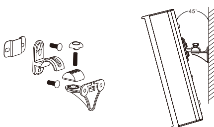
角度調整できるブラケット(0-45° 別売り)
